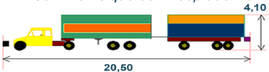
Semirremolque con Acoplado
